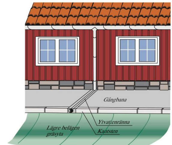
Figur 8. Dagvatten avleds från stuprör i ränna och mot dike eller gräsyta.
