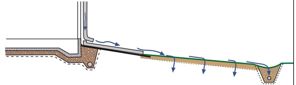
Figur 7. Exempel på hur dagvatten kan avledas med hjälp av stuprörsutkastare och dräneringsstråk. Dräneringsstråket läggs på den egna fastigheten.
