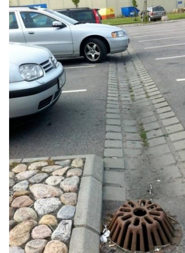
Figur 4. Med små diken vid bilarnas front kan dagvatten avledas ytligt.
