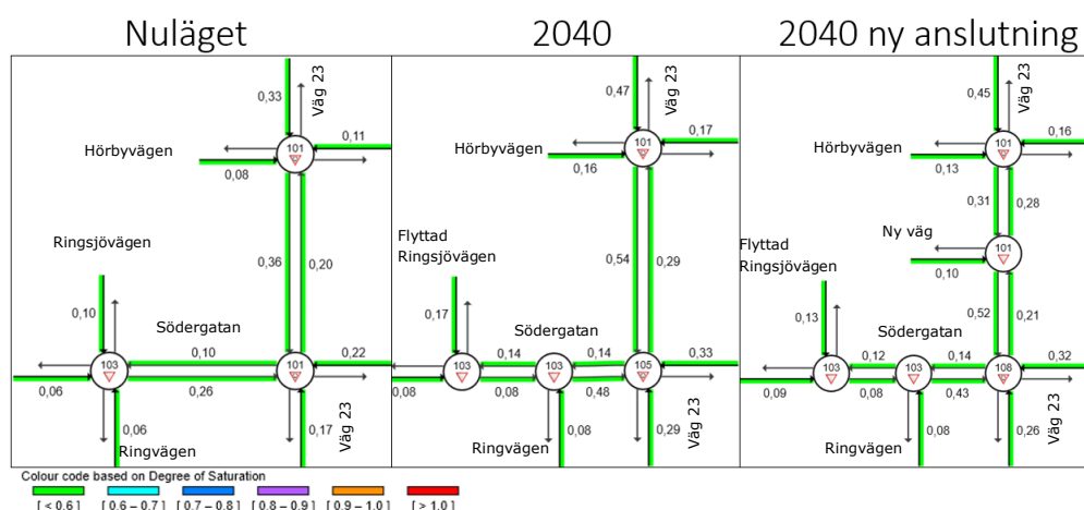
Figur 16 belastningsgrad under morgonens maxtimme för det studerade korsningspunkterna.
