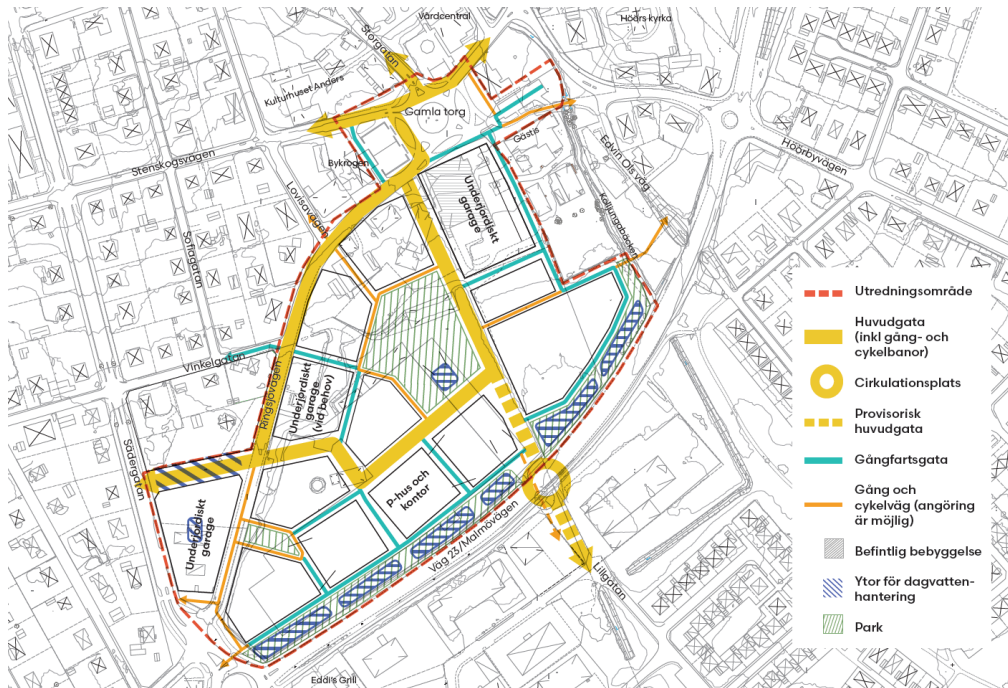
Figur 9 Skiss på intern gatustruktur vid full utbyggnad, bild under bearbetning från Tengbom 2020.
