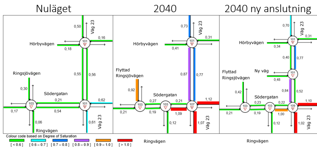
Figur 17 belastningsgrad under eftermiddagens maxtimme för de studerade korsningspunkterna.
