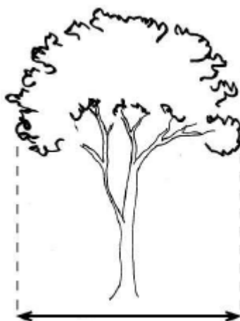
Fig. 4 Trädets droppzon.
